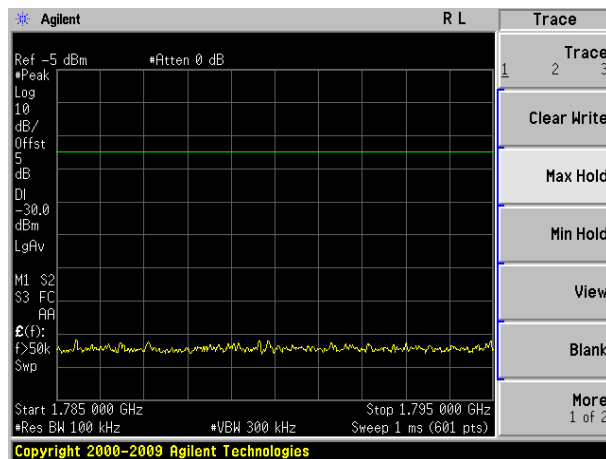
1.785GHz~1.795GHz
