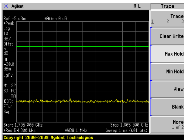
1.795GHz~1.805GHz
