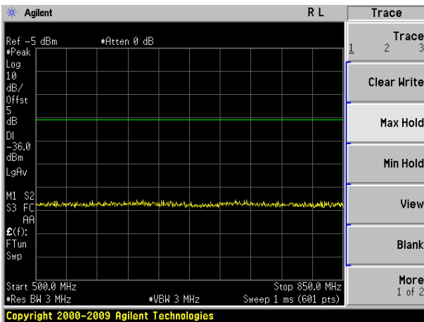
500MHz~850MHz
