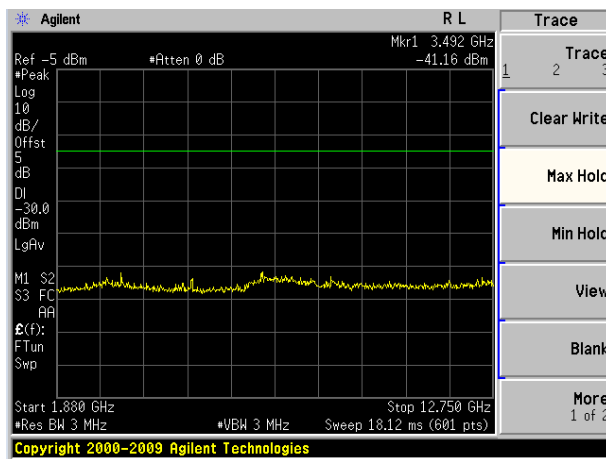
1.88GHz~12.75GHz
