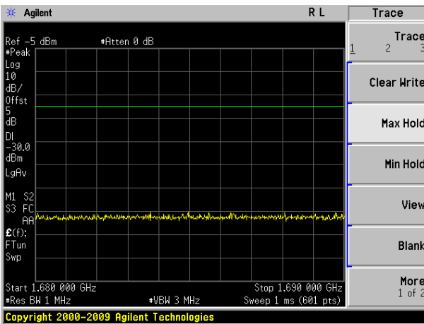
1.68GHz~1.69GHz
