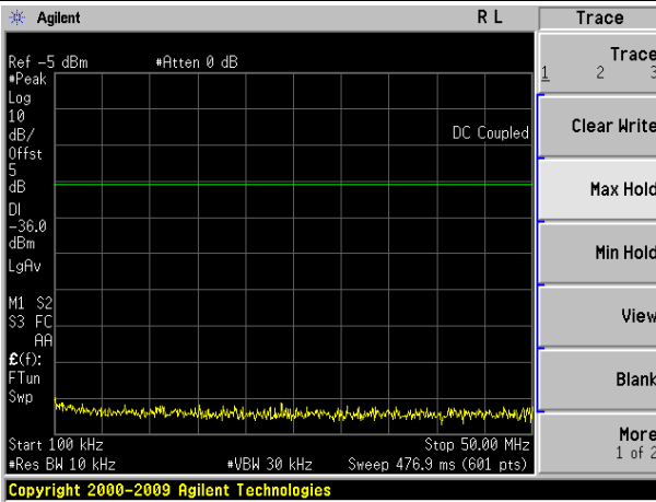
100kHz~50MHz
