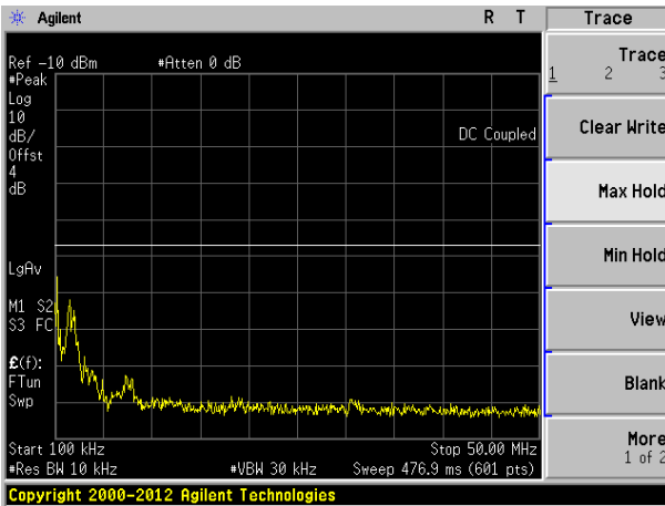
100kHz~50MHz
