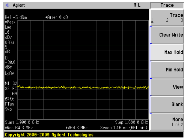
1000MHz~1680MHz
