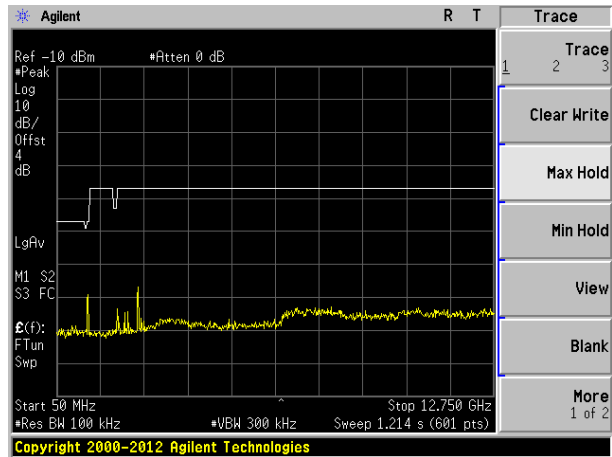
50MHz~12.75GHz
